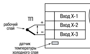
Рисунок 5.13 – Схема подключения термопары
